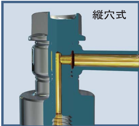
製品内部の穴をオイルが通過します
