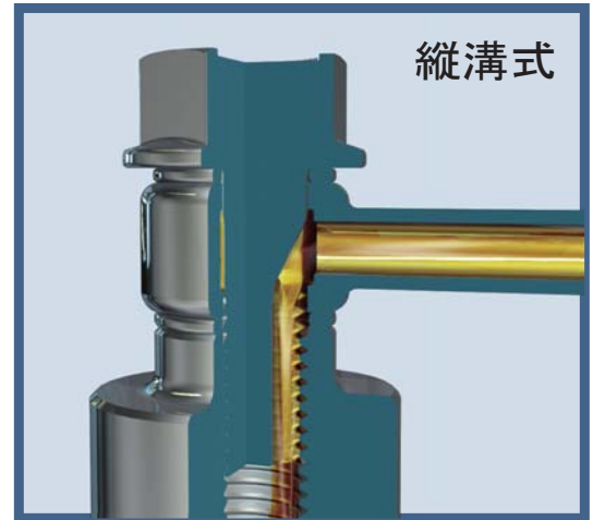
製品外形にある溝にオイルが通過します
